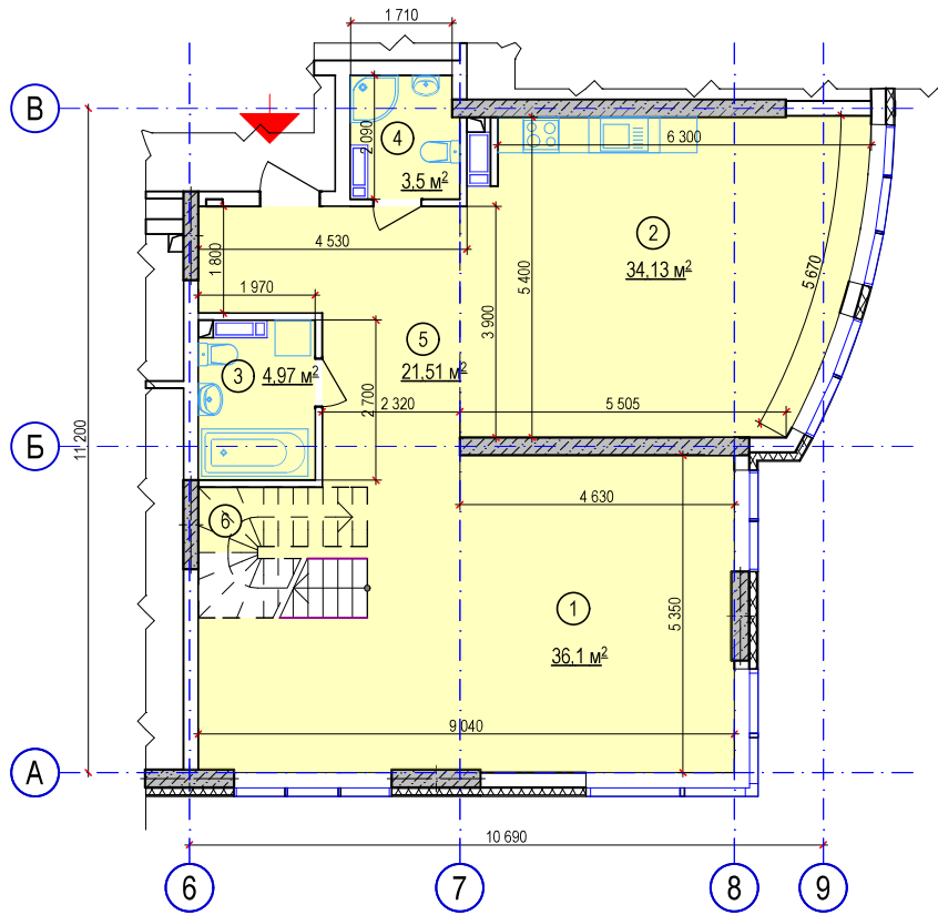
Рівень 1 (23 поверх)
