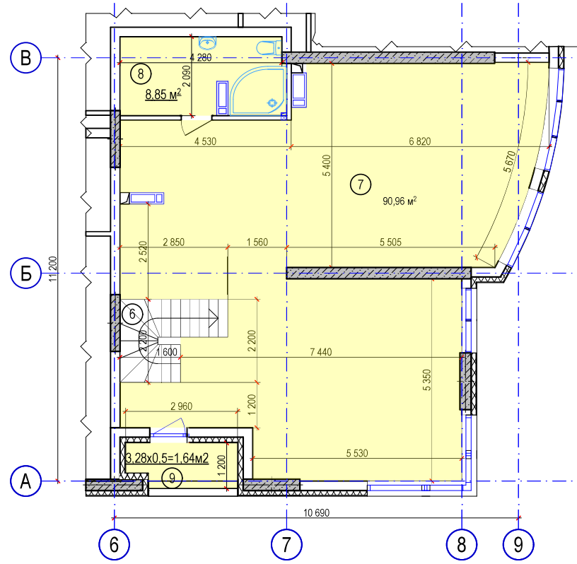
Рівень 2 (24 поверх)
